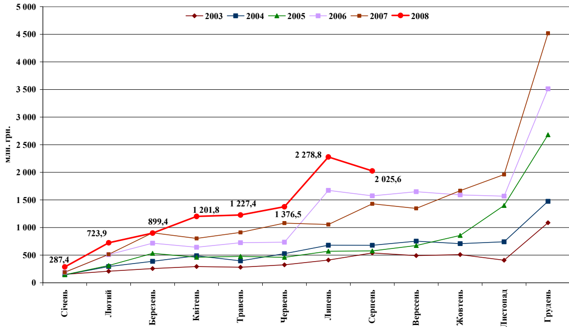
Графік 52
