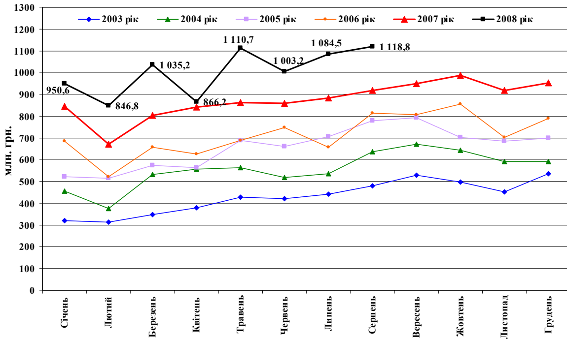
Графік 6
