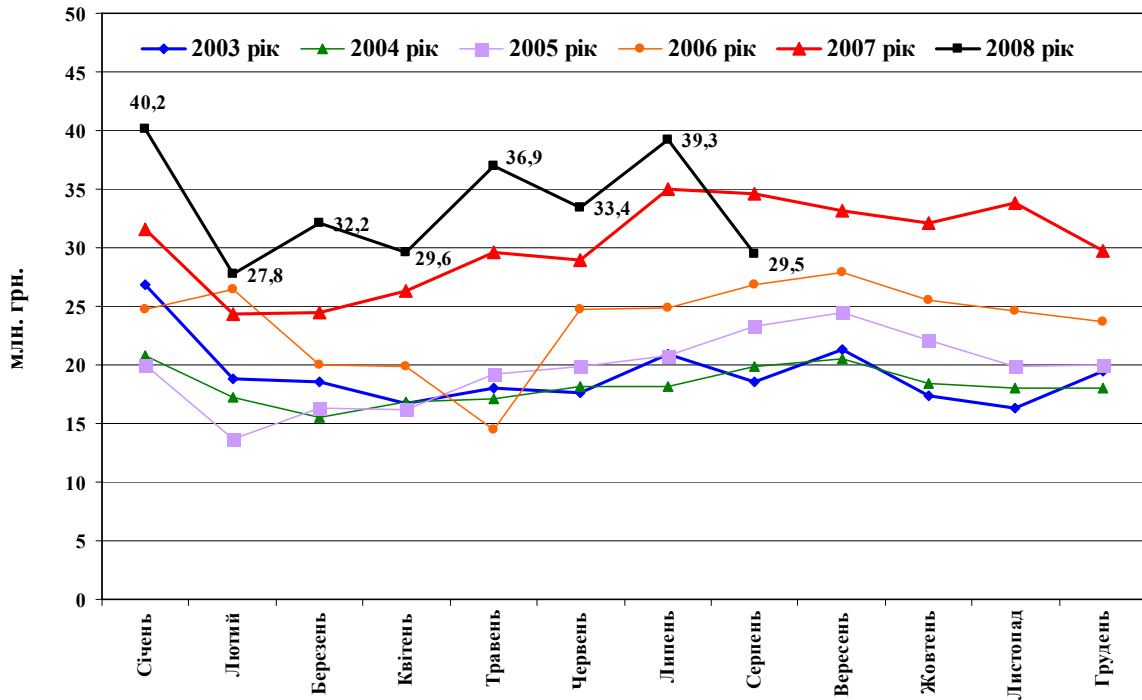
Графік 8
