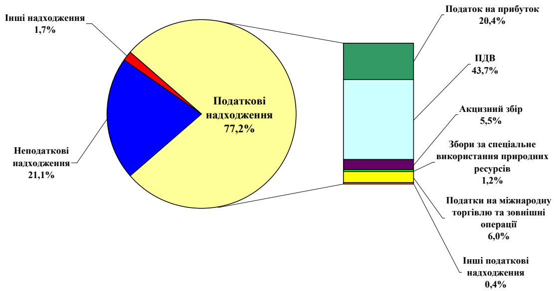
Діаграма 2
