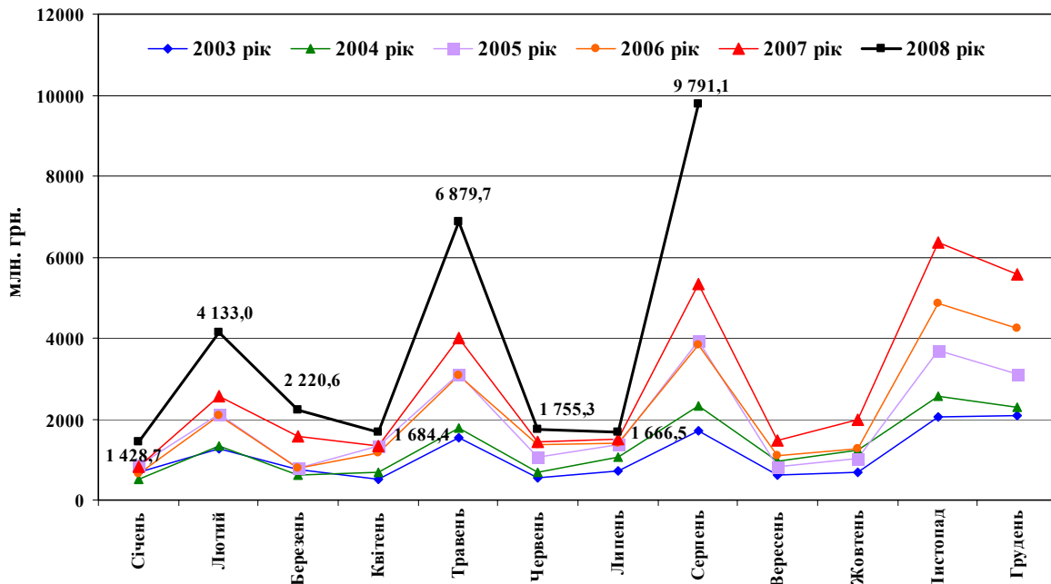
Графік 4
