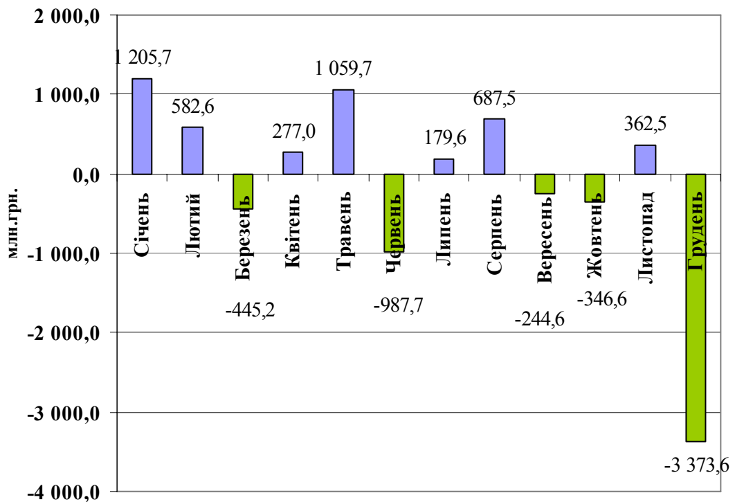
Діаграма 10
