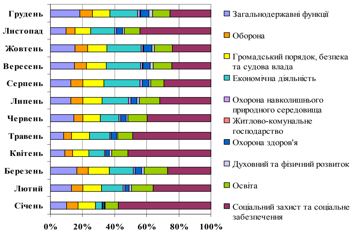
Діаграма 18
