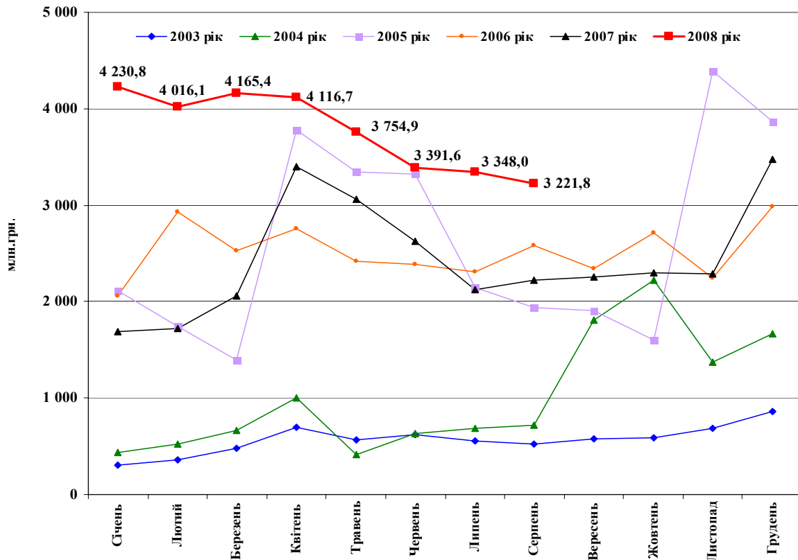
Графік 48
