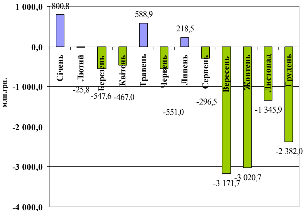
Діаграма 10
